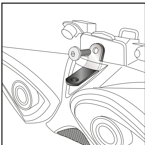
X-förmigen Kunststoffblende - Rückseite x-formed cover - rear side
